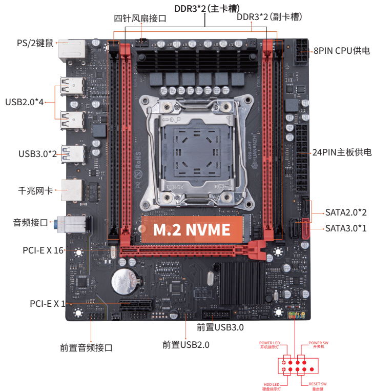
图1-1 X99-4MT主板图解
